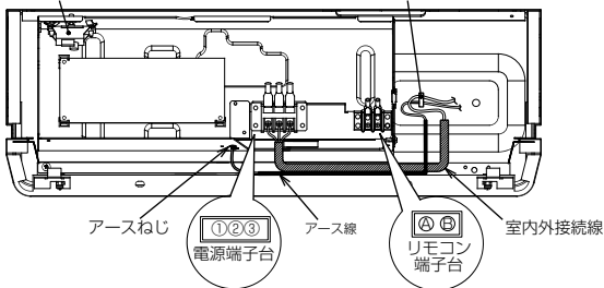
冷媒センサ
