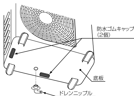
防水ゴムキャップ
